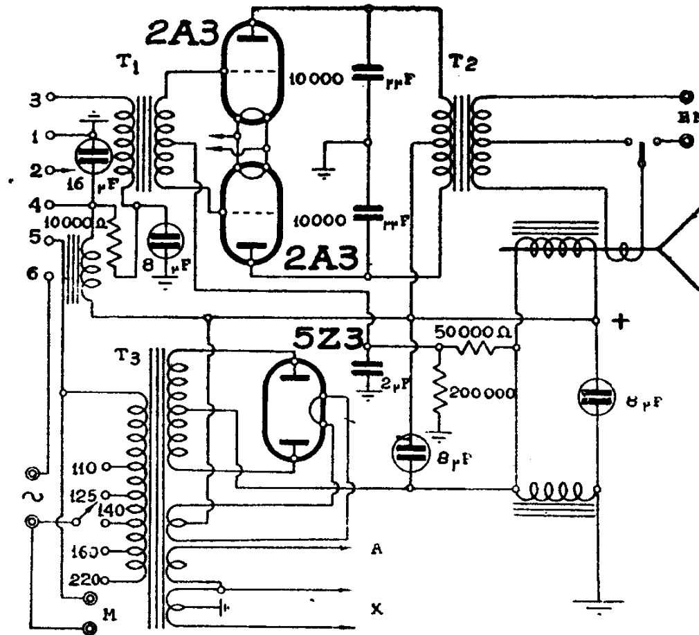
S.A.F.A.R. - MOD. « 73 » - PARTE BF E ALIM.
